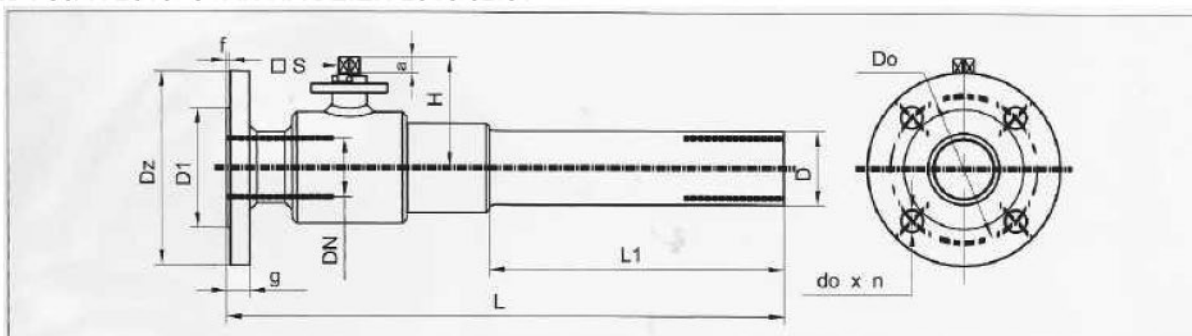
Wymiary podstawowe
